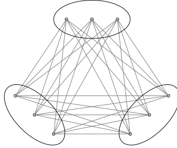
FIGURA 4: El graf extremal de 9 vèrtexs que no conté K_4 .
